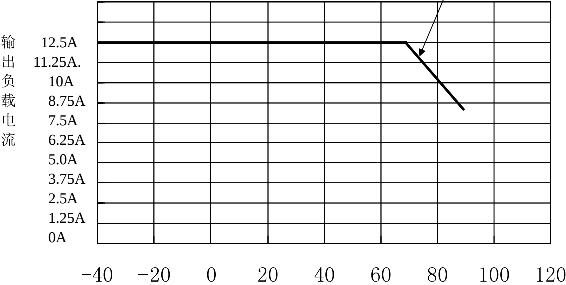
环境温度（℃） （带散热器）温度降额曲线
